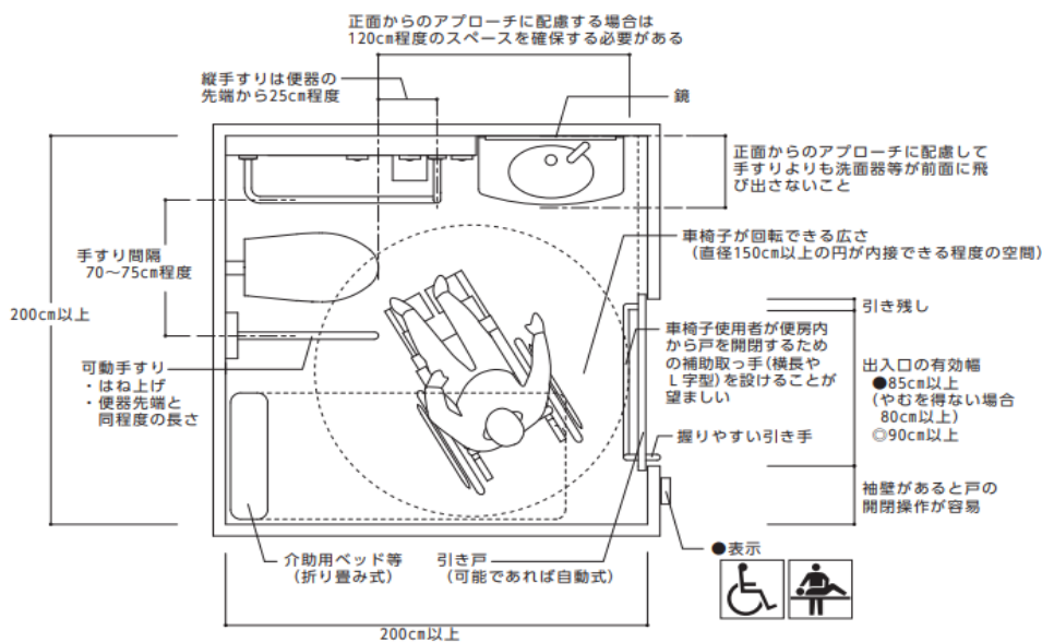
【図8.2】車椅子利用者用便房の例（内法200cm×200cm以上の場合）
